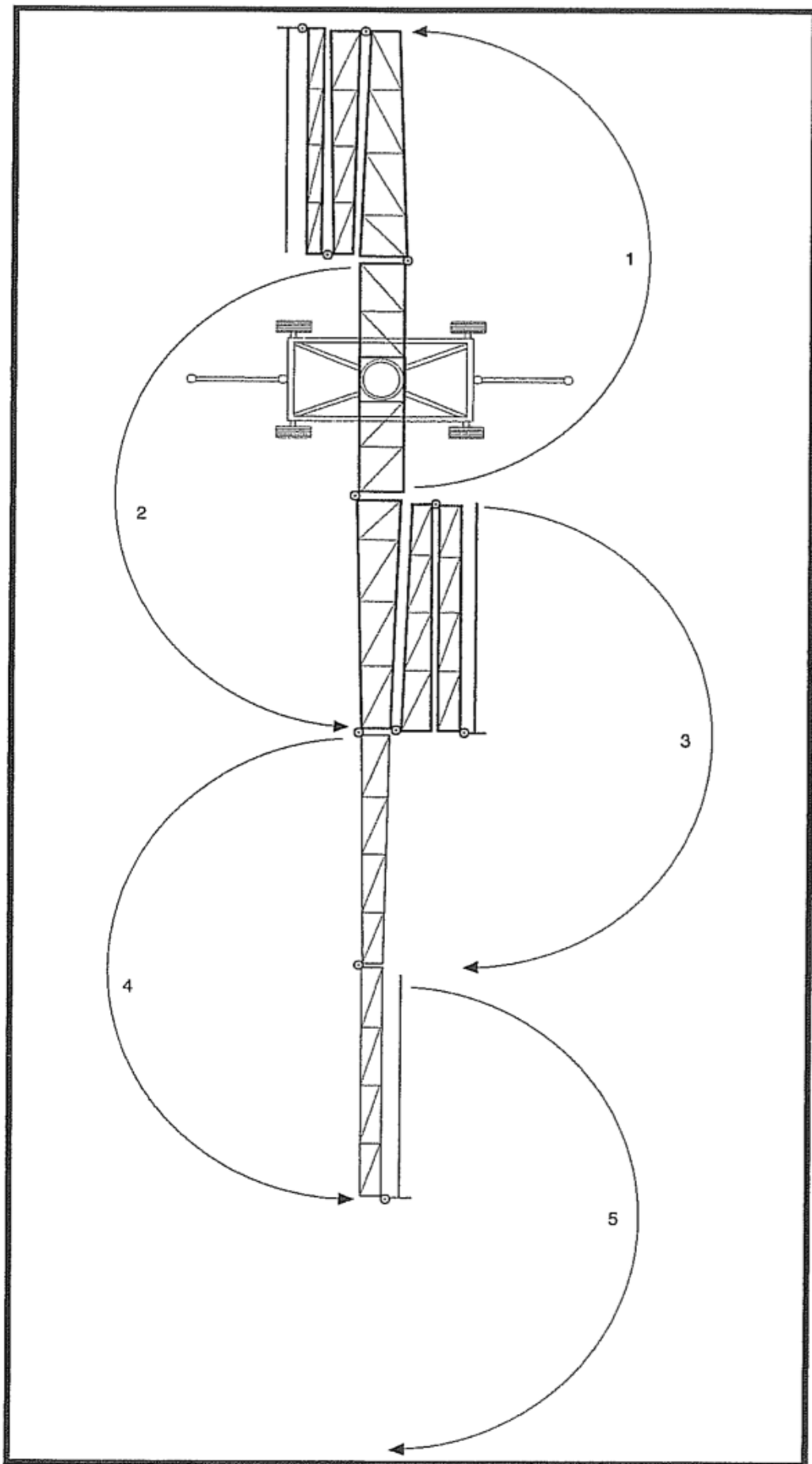
Übersichtsskizze des Aus- und Einklappvorgangs
